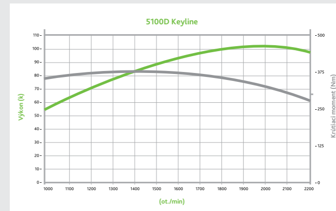
↑ Výkonová charakteristika modelu 5100D Keyline.
